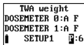
图 10 Setup TWA
